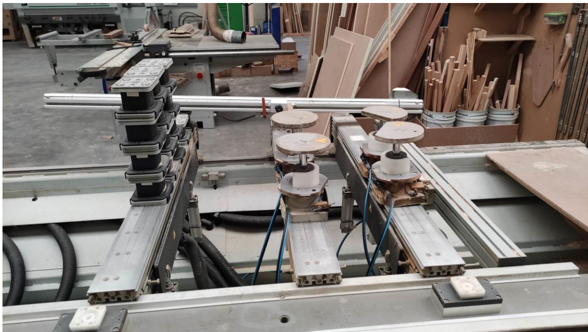
Fot. 16. Stół maszyny z podporami materiału
